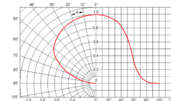
Рисунок 5 Типы КСС
